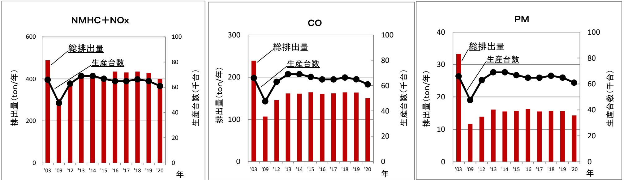
図1. ディーゼルエンジン排出ガス量（2020年）
